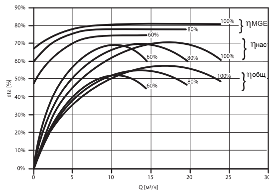
Рис. 3 КПД MGE электродвигателя, насоса и общий КПД E-насоса при скоростях 100%, 80% и 60% от максимальной скорости вращения вала насоса.
