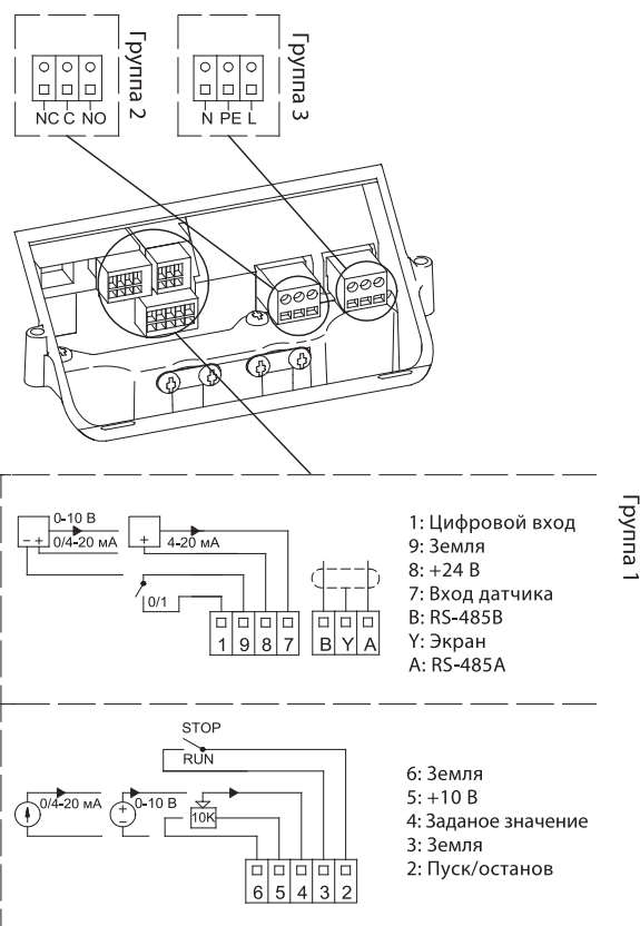
Рис. 35 Схема подключения
